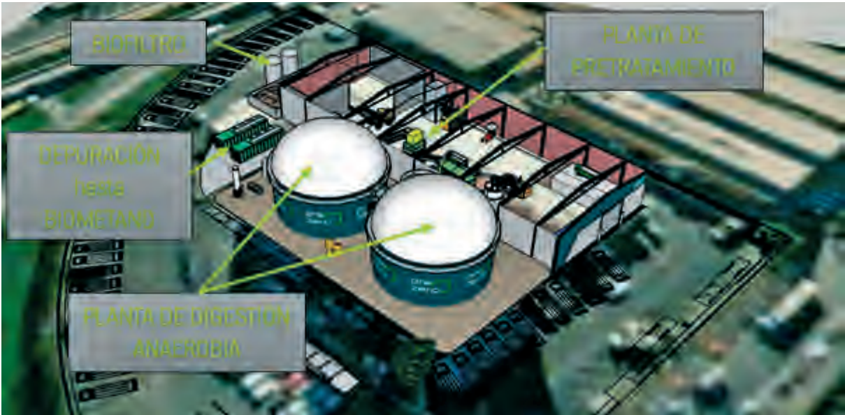
ESQUEMA GRÁFICO DE LA ESTRUCTURA DE LA FUTURA PLANTA DE BIOGÁS, QUE TAMBIÉN PRODUCE DIGESTATO PARA USOS AGRÍCOLAS Y COMPOSTAJE
