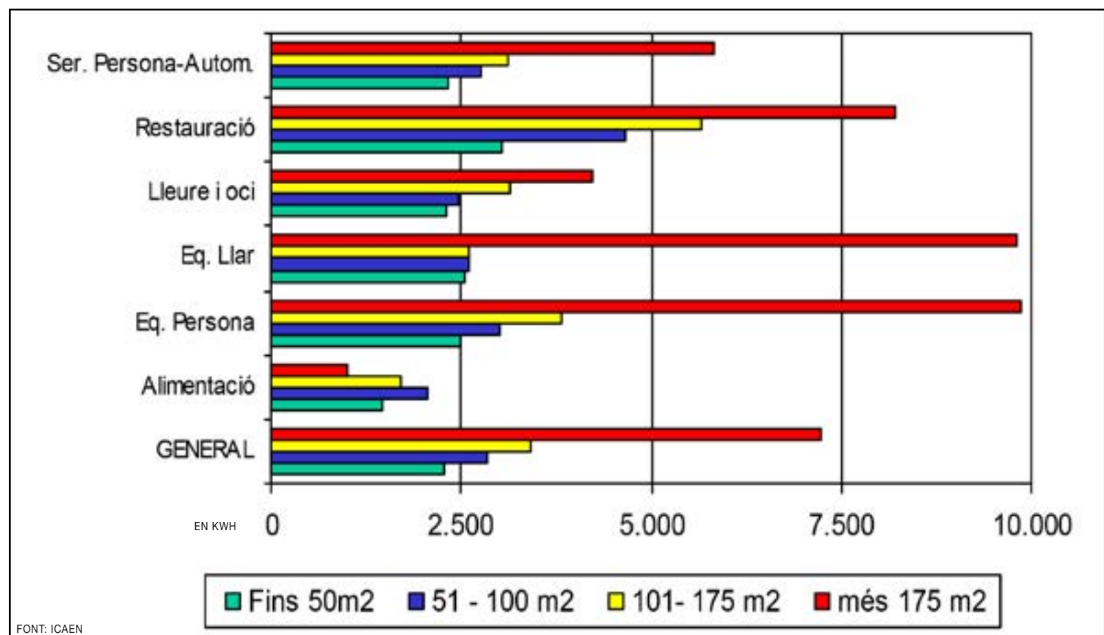
Consum mitjà d'aire condicionat per sectors i dimensió de l'establiment
